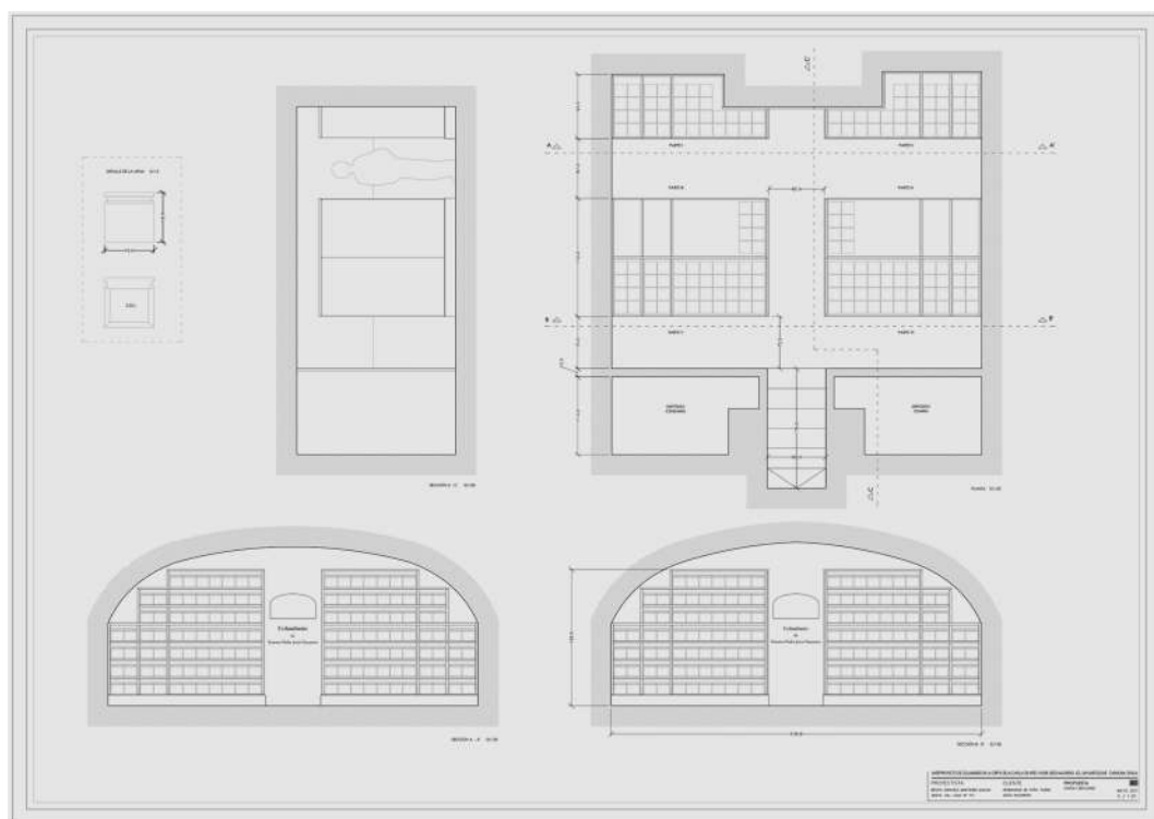
▲ Planos generales del columbario, 2011.
